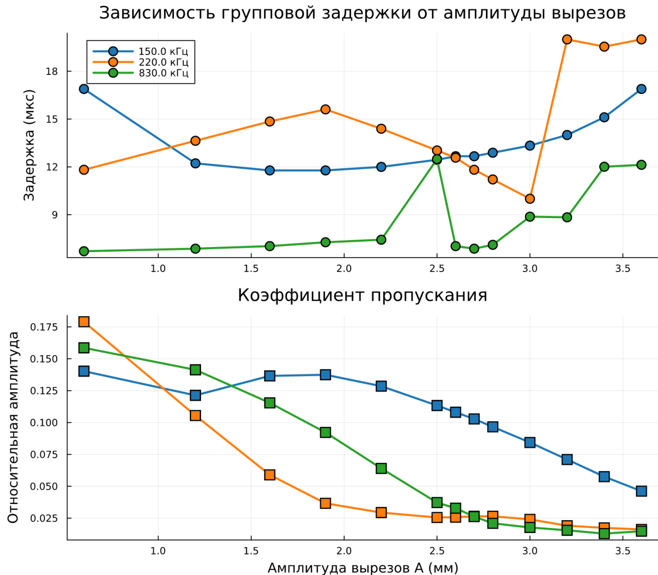
Рис. 3: Рис.3, совмещенные графики задержки и пропускания
