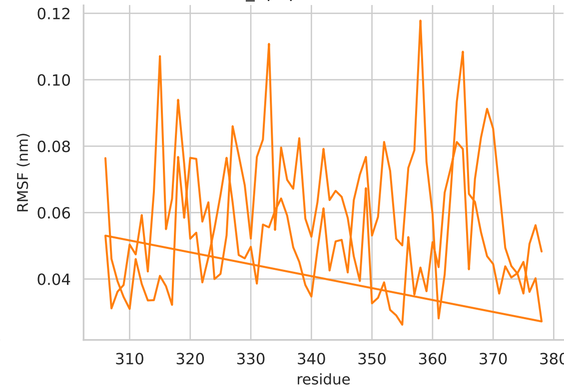
fibril_tip: per-residue RMSF
