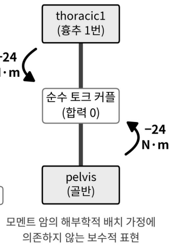
Figure 1. 근골격계 모델과 슈트 모델링. (a) 전신 모델과 슈트 인장 경로, (b) 흉추 1-골반 간 순수 토크 커플, (c) 액추에이터 사양에서 해석 토크 유도.
