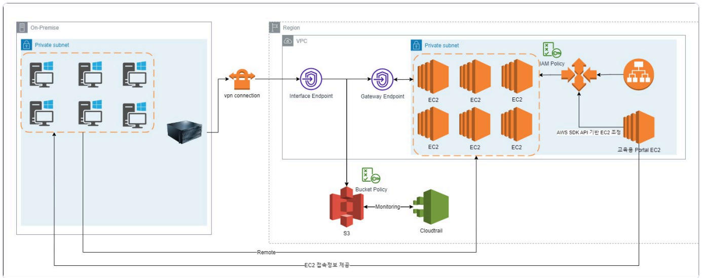
SDP 교육용 AWS 아키텍처 구성도 — 교육용 Portal EC2가 AWS SDK API로 학생별 EC2를 조정
