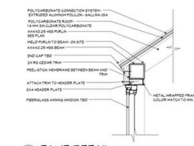
5 EAVE DETAIL A3.1 SCALE: 1 1/2" = 1'-0"
