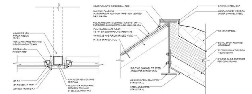
9 STEEL COLUMN DETAIL A3.1 SCALE: 1 1/2" = 1'-0"
