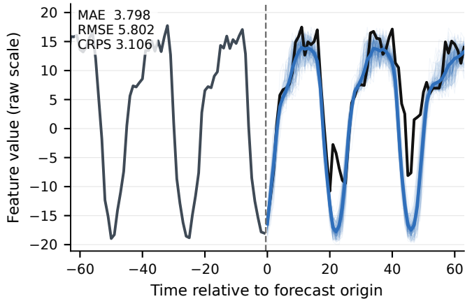
ETTh — Diffusion-TS
