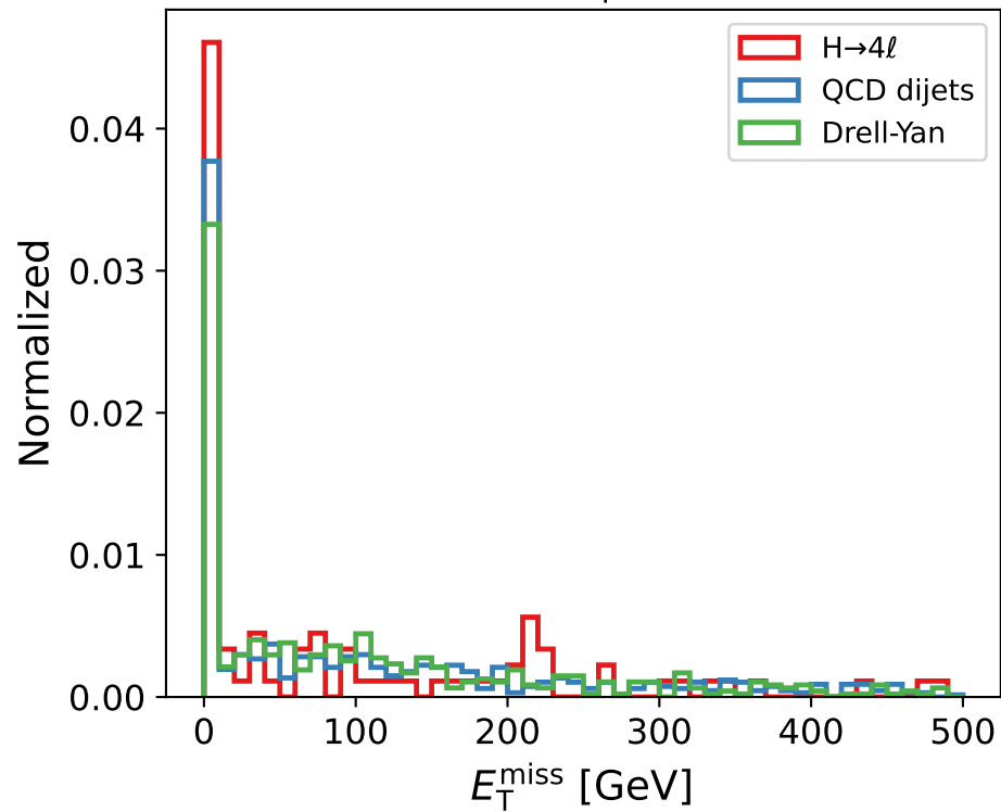
(b) E_T^{\text{miss}}
