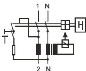
2 Pole RCCB
