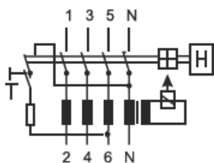
4 Pole RCCB
