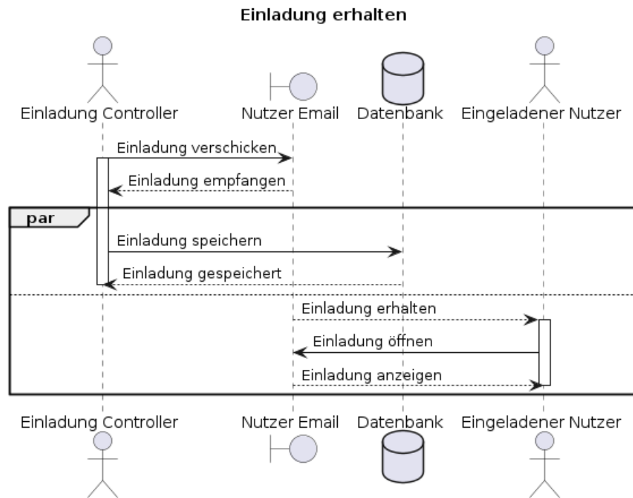
Figure 2: F007_einladungErhalten_seq.png
