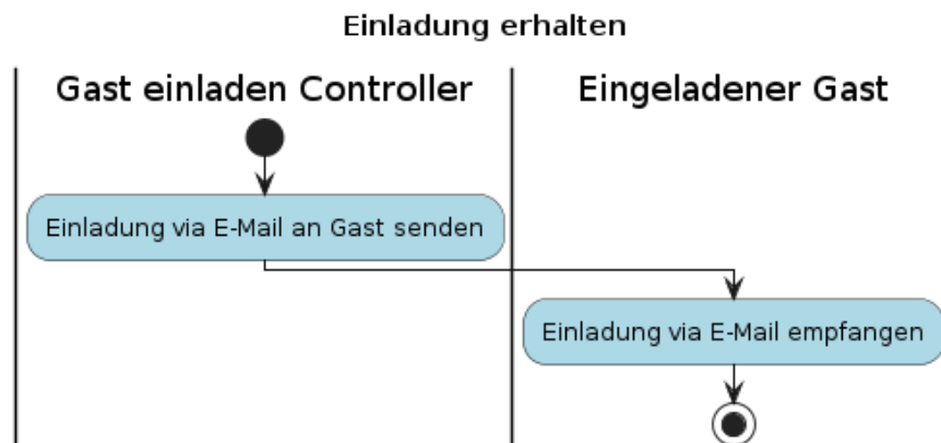
Figure 1: F007_einladungErhalten_act.png
