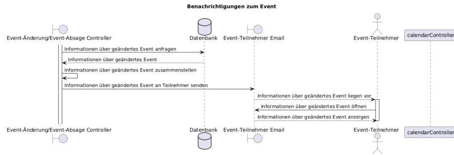
Figure 2: F017_BenachrichtigungenZumEvent_seq.png
