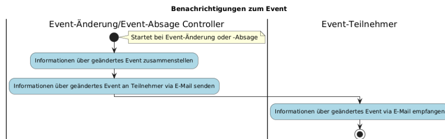
Figure 1: F017_BenachrichtigungenZumEvent_act.png
