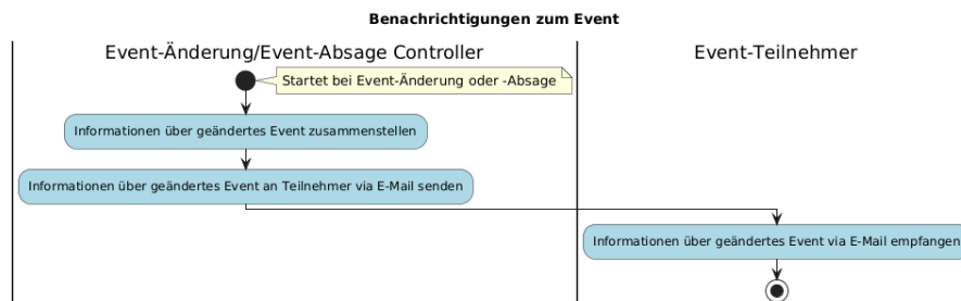
Figure 1: F017_BenachrichtigungenZumEvent_act.png
