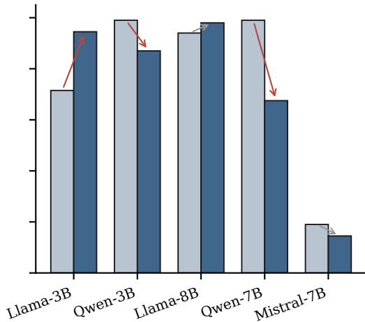
Crescendo
