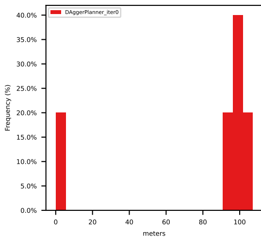
p90_ego_expert_L2_error
