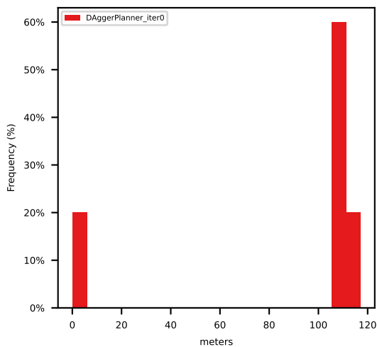
p90_ego_expert_L2_error
