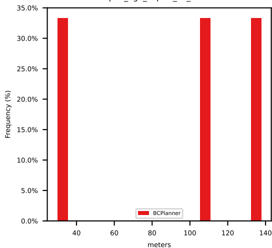
p90_ego_expert_L2_error
