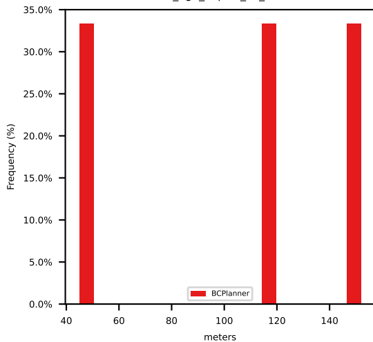
p90_ego_expert_L2_error
