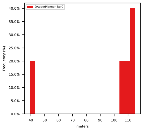
p90_ego_expert_L2_error
