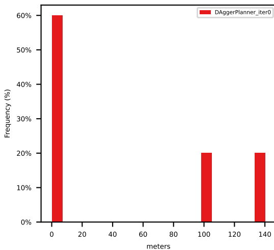
p90_ego_expert_L2_error
