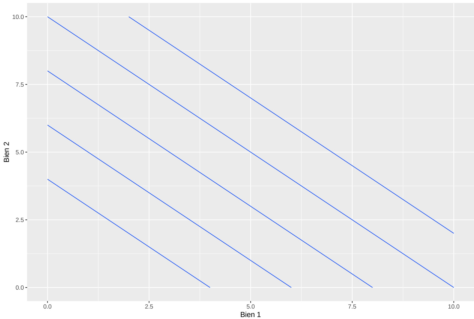
Substituts parfaits ( U = x_1 + x_2 )
