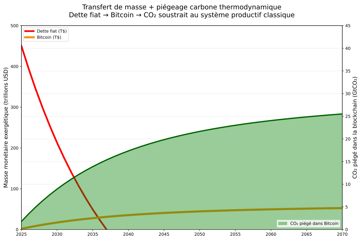
FIGURE 8 – Évolution simulée 2025–2070 (paramètres centraux : \alpha = 0,065 , \beta = 0,50 ). Courbe rouge : valeur exergétique du système dette-fiat. Courbe orange : capitalisation Bitcoin. Remplissage vert : CO 2 intégré à la blockchain (GtCO 2 ).
