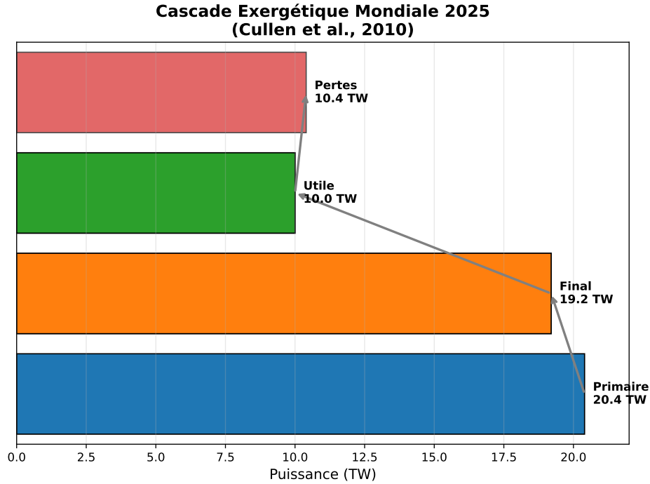
FIGURE 3 – Cascade exergétique mondiale 2025. Primaire (20,4 TW) → Final (19,2 TW, \eta = 94\% ) → Utile (10,0 TW, \eta = 52\% ) → Pertes (10,4 TW) [8].
