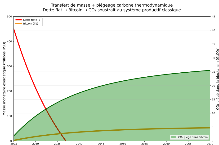
FIGURE 9 – Évolution simulée 2025–2070 (paramètres centraux : \alpha = 0,065 , \beta = 0,50 ). Courbe rouge : valeur exergétique du système dette-fiat. Courbe orange : capitalisation Bitcoin. Remplissage vert : CO 2 intégré à la blockchain (GtCO 2 ).
