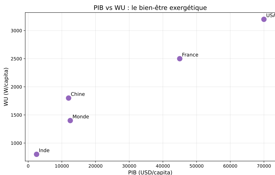
FIGURE 10 – Corrélation WU vs PIB (2025–2050). Cette projection modélisée illustre le dé-couplage exergétique-monétaire . Le WU est piloté par l'efficacité ( \eta ), tandis que le PIB est maintenu par l'inflation et la dette. La croissance future de la société efficace est caractérisée par l'inégalité WU \gg PIB .
