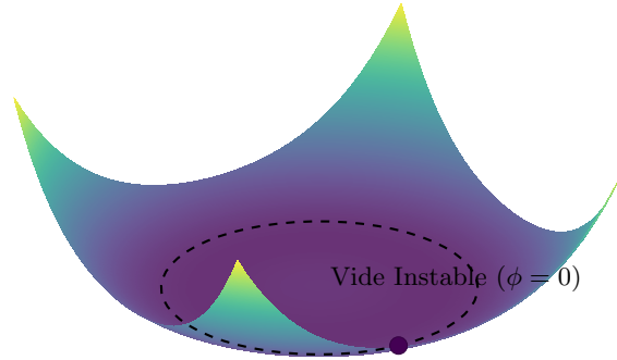
Figure 3 – Le Potentiel de Consensus. Le système roule spontanément de l'origine instable (sécurité nulle) vers la vallée stable \phi_0 (hashrate d'équilibre), définie par l'équilibre entre l'incitation (a) et le coût (b).
