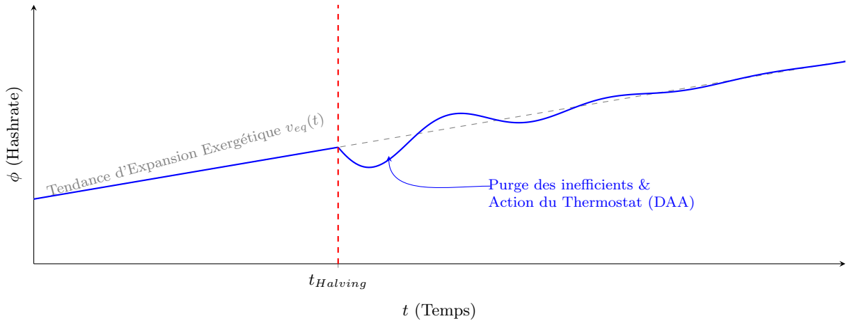
Figure 5 – Trempe sur Fond Non-Stationnaire. Le paramètre d'ordre \phi est soutenu par une croissance séculaire (chasse à l'exergie). Le Halving impose une perturbation abrupte. L'inertie des mineurs et l'intervention du thermostat (DAA) créent un plateau ou un creux transitoire (relaxation amortie) avant que la tendance haussière ne reprenne.
