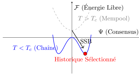
Figure 2 – Brisure de Symétrie dans le Consensus. À haute température effective (travail nul), l'énergie libre \mathcal{F} possède un seul minimum à \Psi = 0 (Désordre/Sybil). En dessous de la température critique (travail positif), le potentiel bifurque. Le système doit spontanément "rouler" dans l'un des vides stables (un historique spécifique), brisant ainsi la symétrie. Revenir à l'autre vide (Double Dépense) nécessite de surmonter la barrière de potentiel \Delta \mathcal{F} , qui croît avec la profondeur de confirmation.
