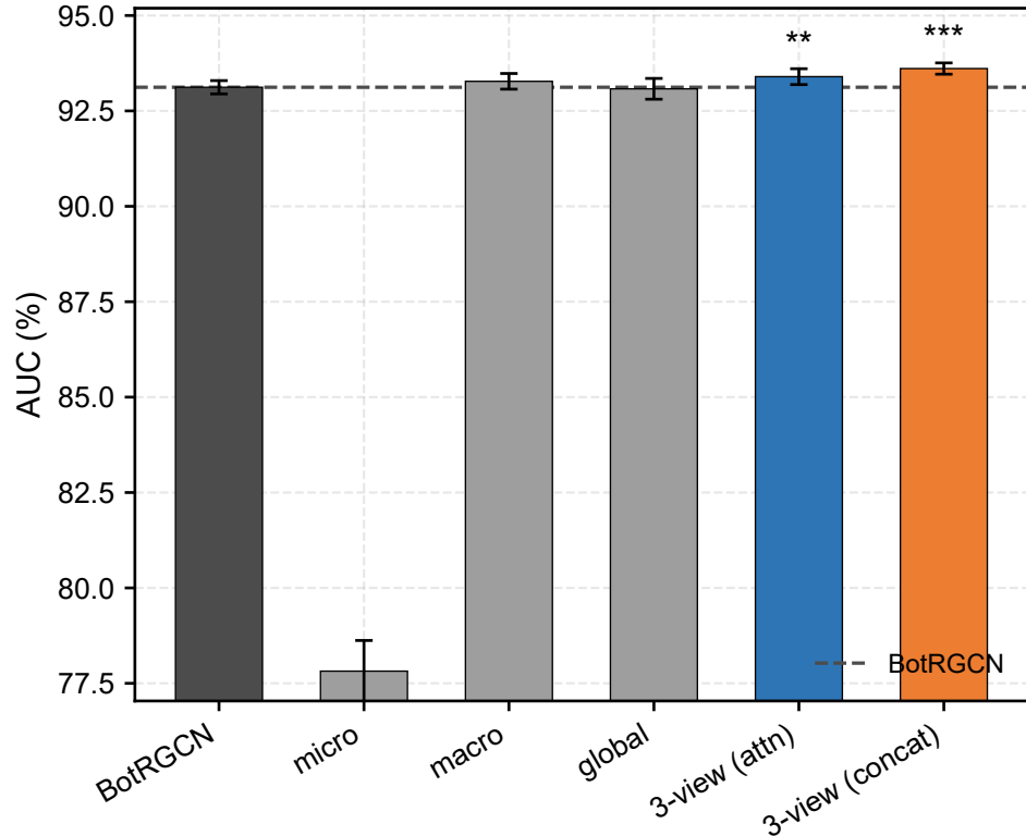
Twibot-20 Ablation (AUC)
