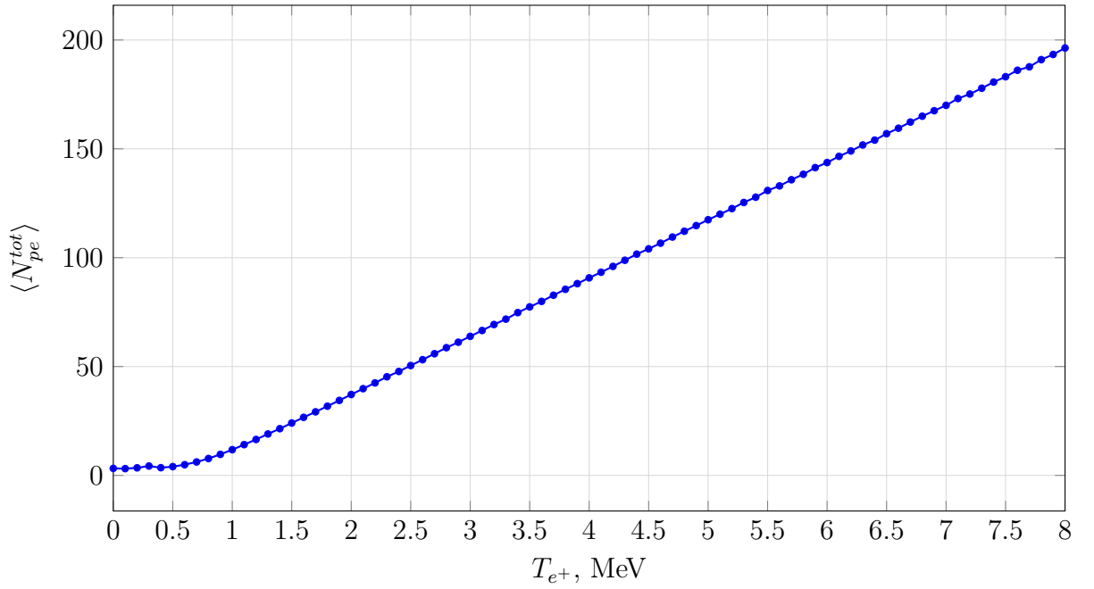
Рисунок 3 — Зависимость среднего числа фотоэлектронов \langle N_{pe}^{tot} \rangle от кинетической энергии позитрона при условии N_{fired} \geq 3 (моноэнергетические позитроны на равномерной сетке T_{e+} , 2 \times 10^4 событий на точку).
