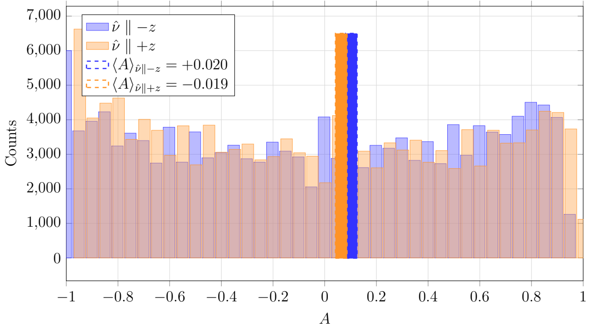
Рисунок 5 — Распределение событийной асимметрии A для prompt-сигнала IBD при противоположных направлениях антинейтрино вдоль оси z (модель Vogel–Beacom, без нейтрона, N_{fired} \geq 3 , \sim 1.4 \cdot 10^5 событий на направление после триггера). Пунктирные вертикальные линии обозначают средние \langle A \rangle .
