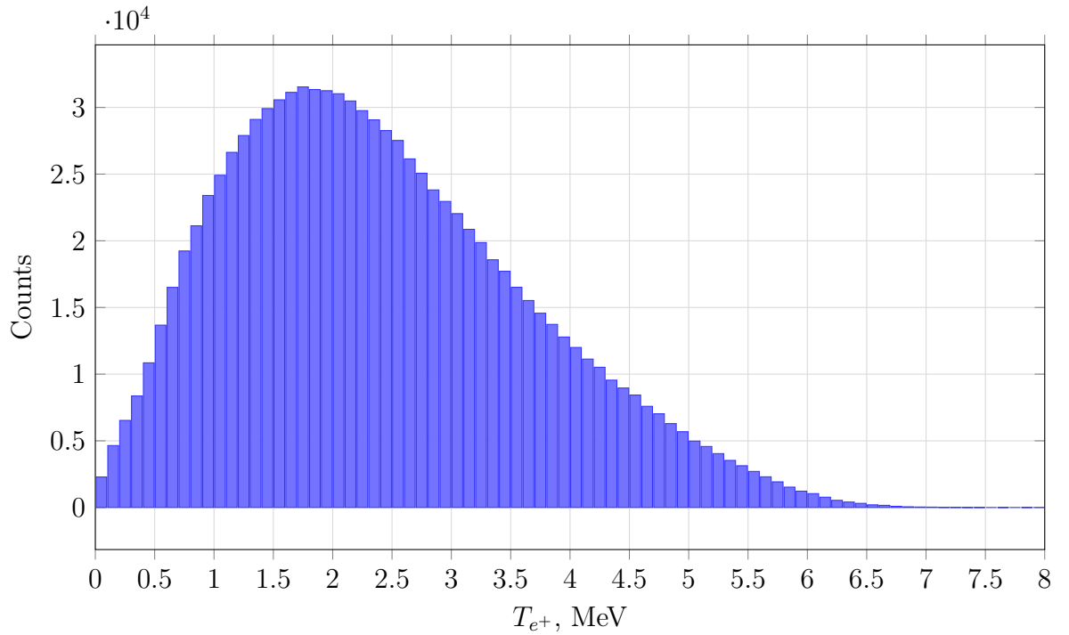
Рисунок 2 — Зарегистрированный спектр кинетической энергии позитронов в реакции IBD при условии N_{fired} \geq 3 (98.8% от 10^6 сгенерированных событий).
