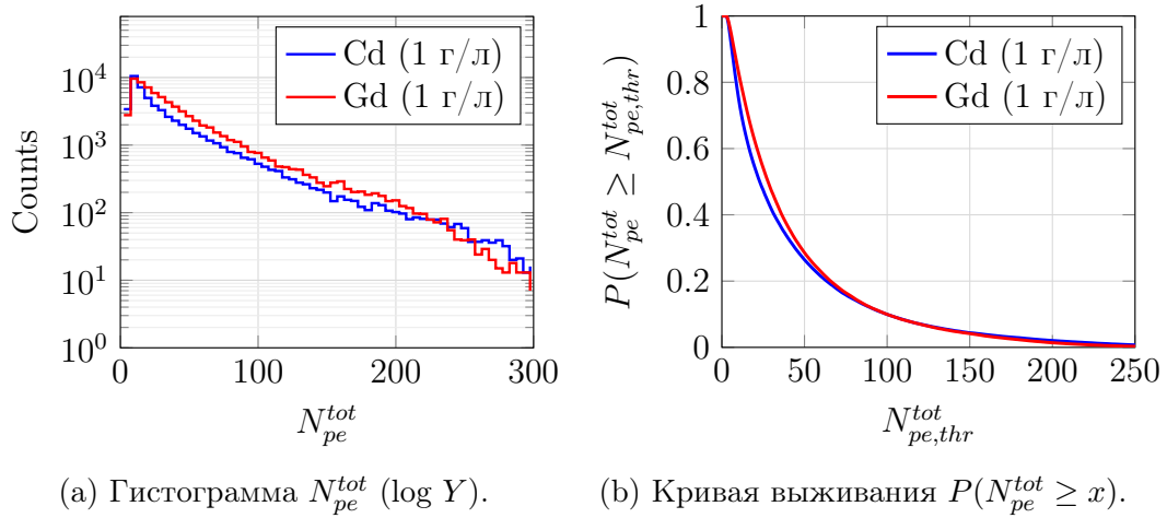
Рис. 4: Сравнение отклика детектора на захват теплового нейтрона для допантов Cd и Gd при концентрации 1 г/л и условии N_{fired} \geq 3 ( 10^5 событий каждой конфигурации). Слева — гистограмма N_{pe}^{tot} в логарифмическом масштабе. Справа — кривая выживания: кривая Gd лежит выше Cd на всём диапазоне световых выходов.
