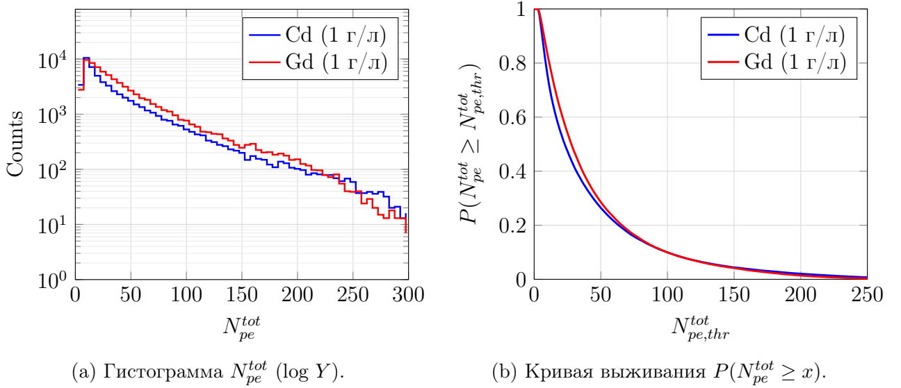
Рис. 4 – Сравнение отклика детектора на захват теплового нейтрона для допантов Cd и Gd при концентрации 1 г/л и условии N_{fired} \geq 3 ( 10^5 событий каждой конфигурации). Слева — гистограмма N_{pe}^{tot} в логарифмическом масштабе. Справа — кривая выживания: кривая Gd лежит выше Cd на всём диапазоне световых выходов.
