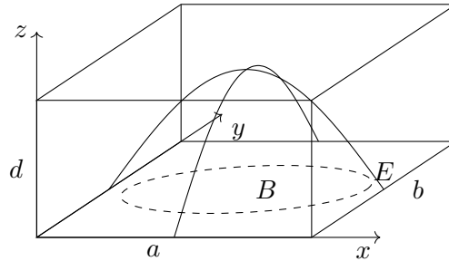
Figura 7.7.: Campi all'interno della cavità
