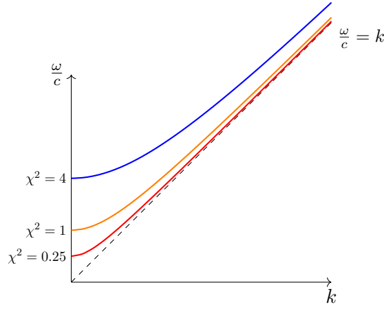
Figura 7.10.: Grafico delle relazioni di dispersione per vari valori di \chi^2 .
