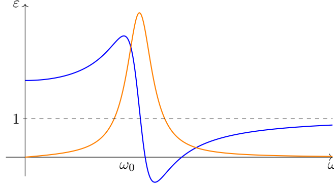
Figura 10.2.: Andamento di \varepsilon_1 e \varepsilon_2 .
