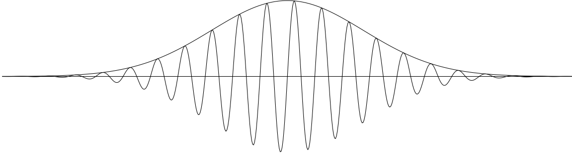
Figura 7.8.: Pacchetto d'onda gaussiano
