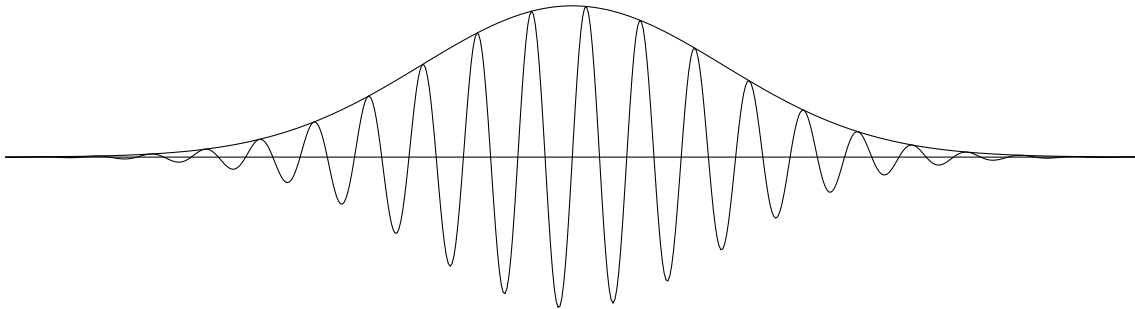
Figura 7.9.: Pacchetto d'onda gaussiano
