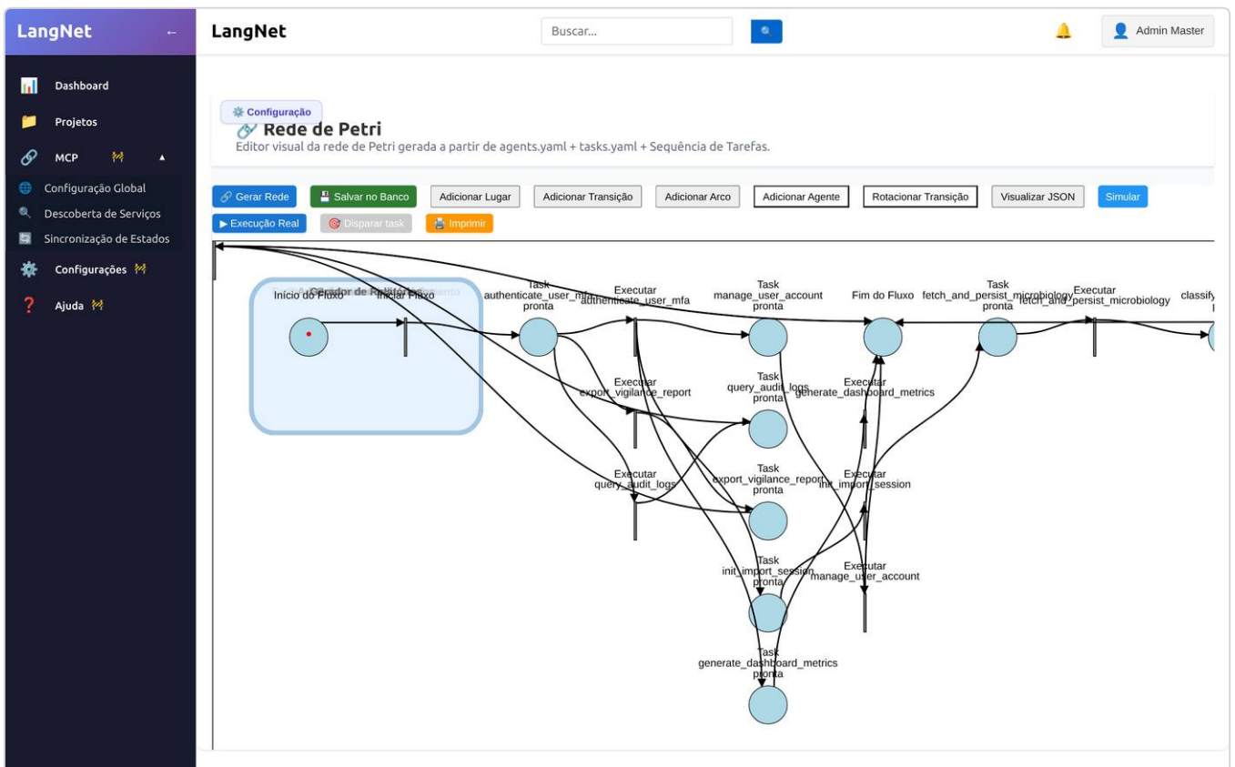
85_petri_net.png
