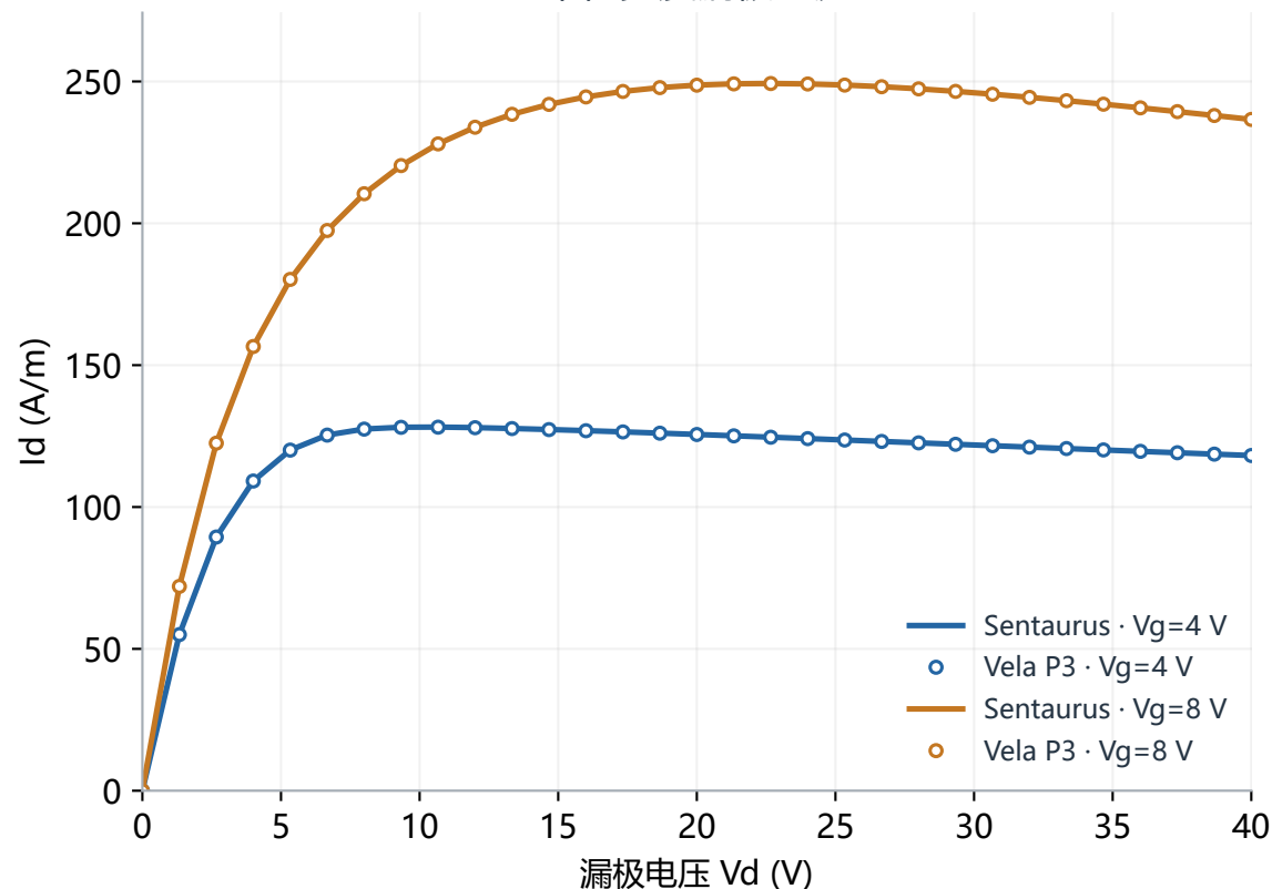
单位宽度漏极电流
