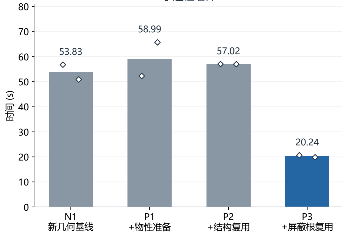
子进程墙钟
