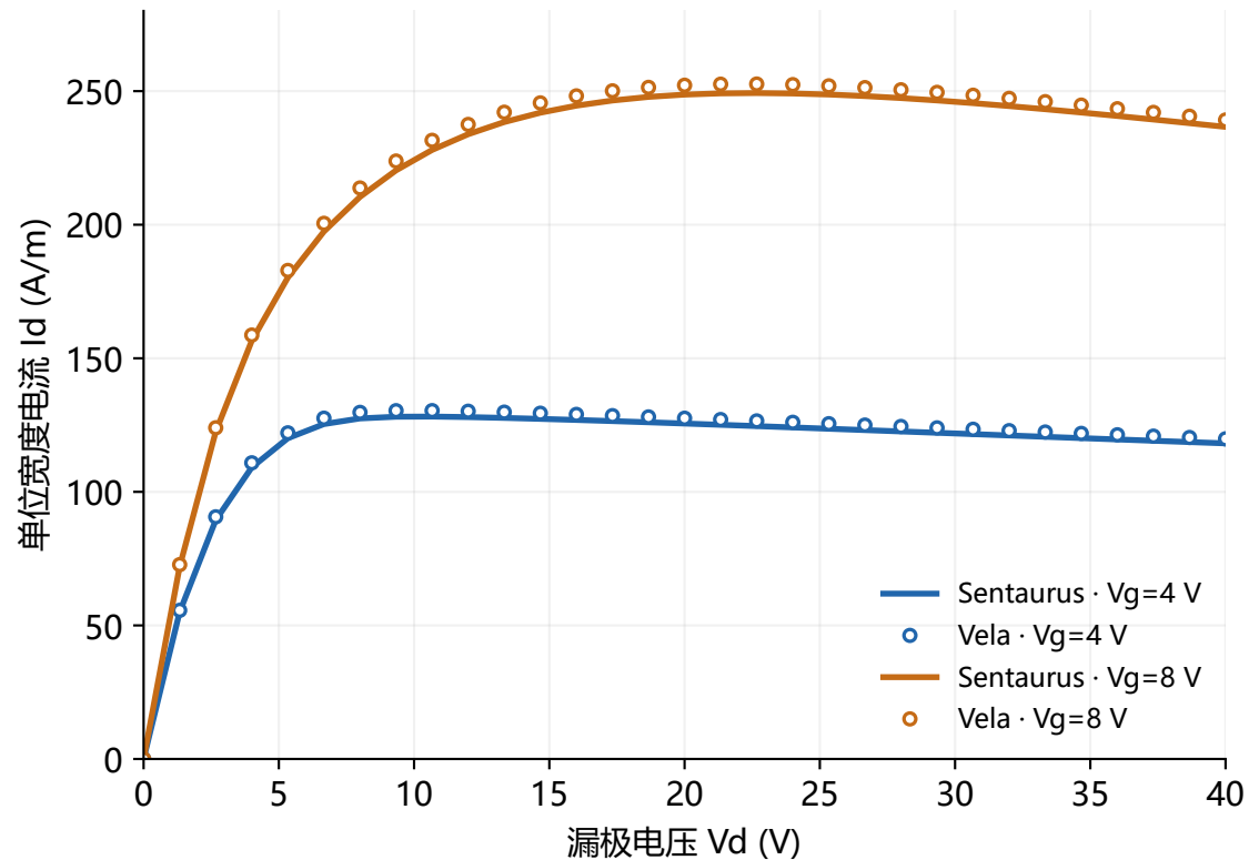
漏极电流
