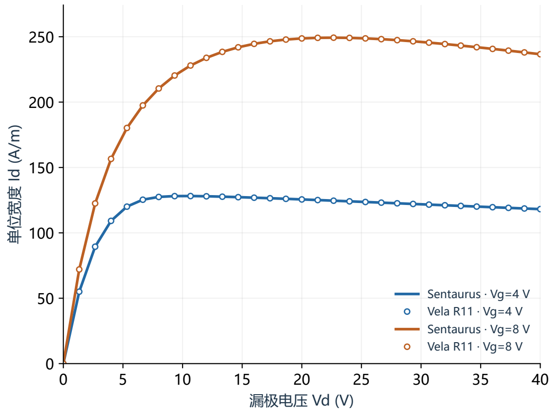
D0 漏极电流
