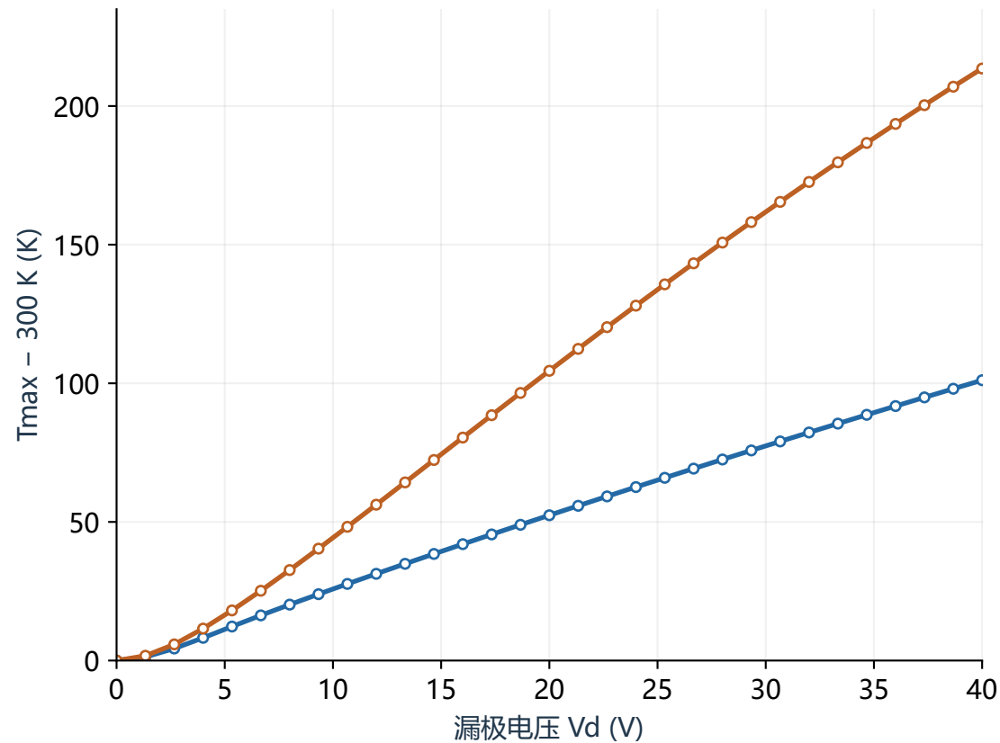
全域峰值温升
