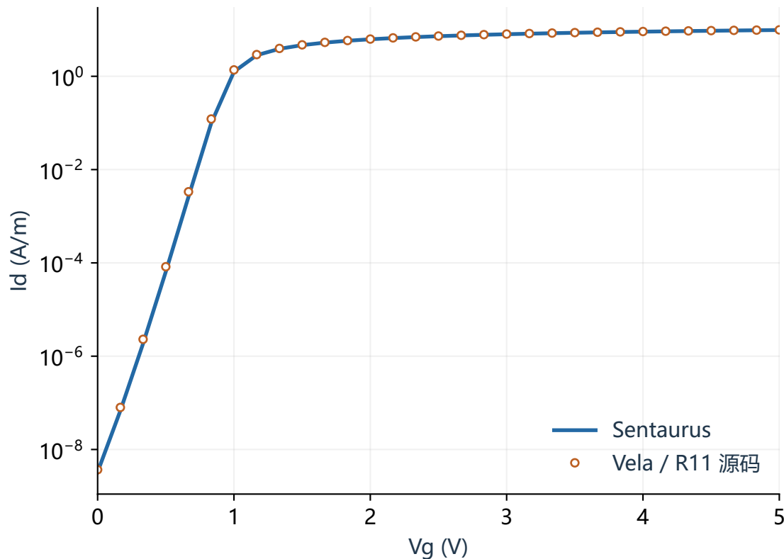
对数坐标：亚阈值区
