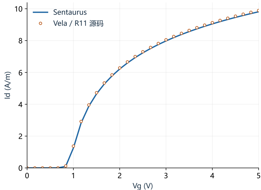
线性坐标：强反型区
