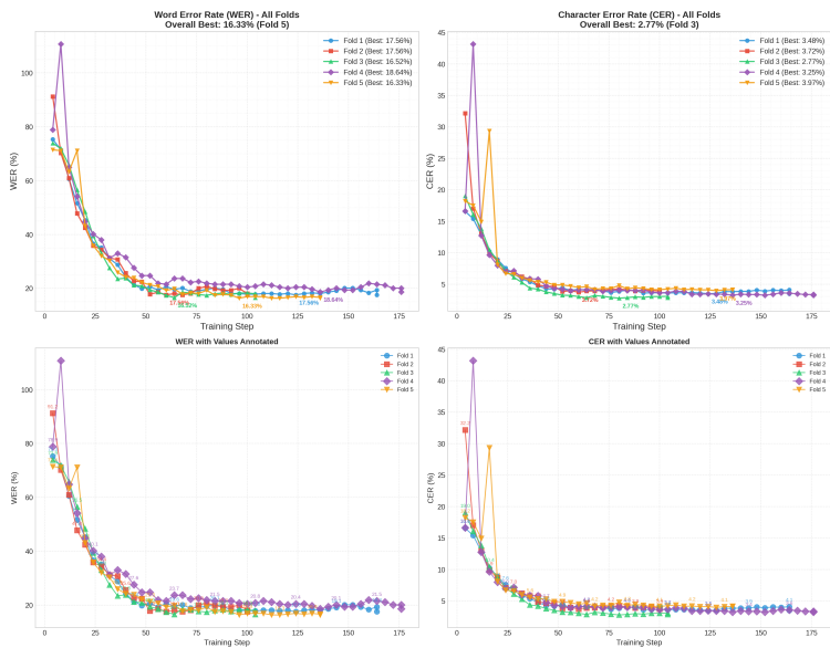
Gambar 4.3 Perkembangan WER dan CER — Strategi LoRA
