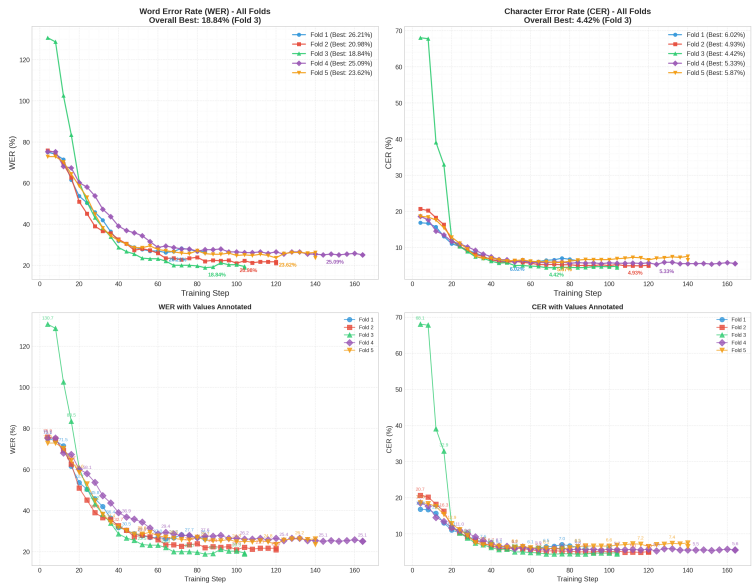
Gambar 4.2 Perkembangan WER dan CER Selama Evaluasi
