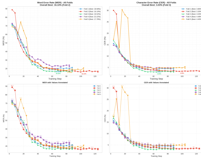
Gambar 4.2 Perkembangan WER dan CER Strategi Freeze Encoder (FE-9)
