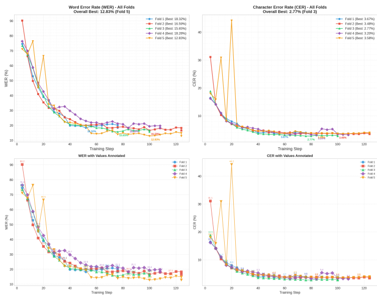
Gambar 4.4 Perkembangan WER dan CER Strategi LoRA (L-9)
