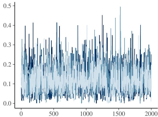
sigma_width
