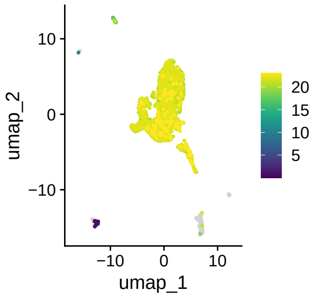
cnv
