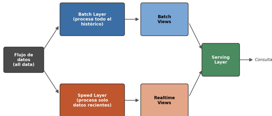
Figura 2.2. Arquitectura Lambda: las capas batch y speed se fusionan en la capa de servicio. Elaboración propia a partir de [2], [3].
