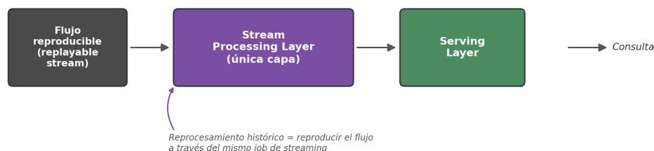
Figura 2.3. Arquitectura Kappa: una única capa de streaming, con reprocesamiento histórico mediante reproducción del flujo. Elaboración propia a partir de [4].
