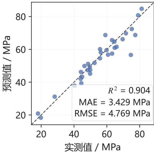
(a) 抗压强度预测值与实测值对比
