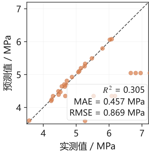
(b) 抗折强度预测值与实测值对比
