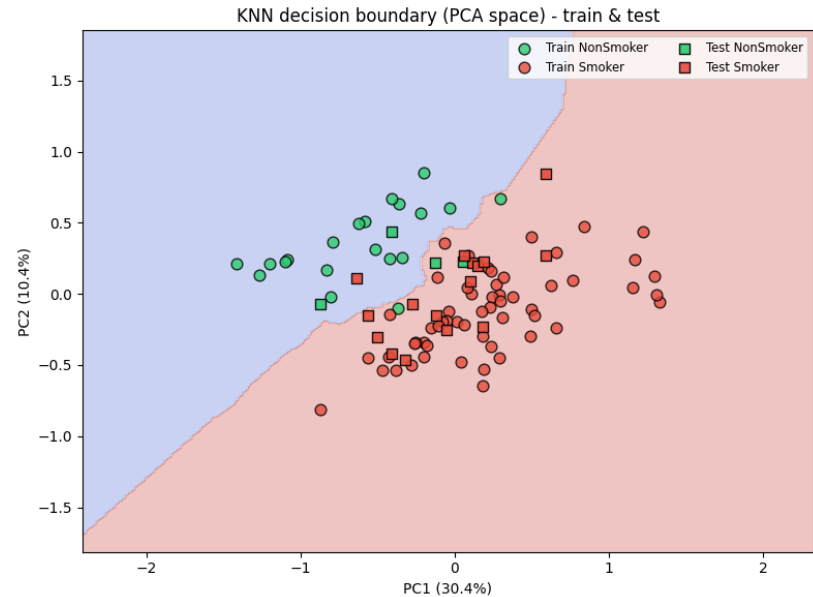
PCA projekcia
