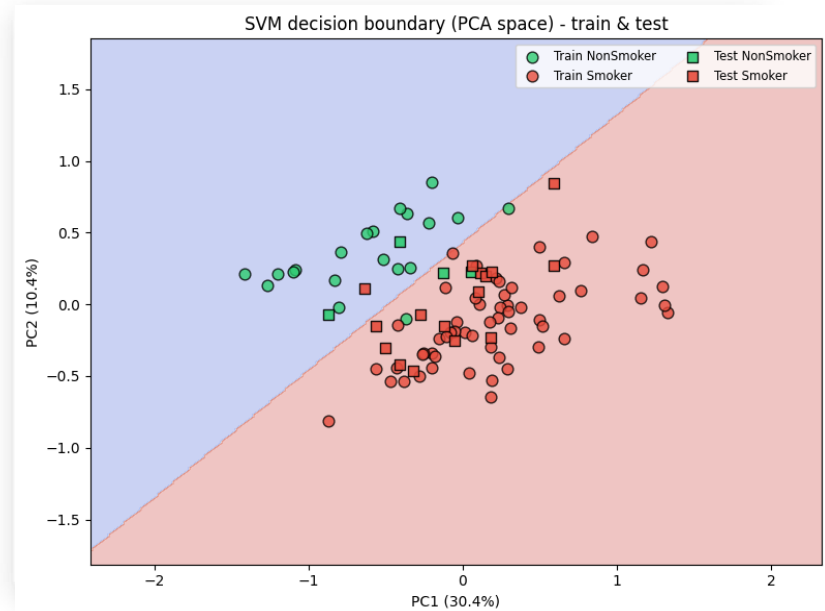
PCA projekcia
