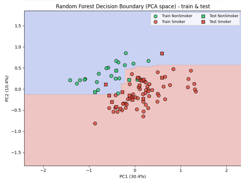
PCA projekcia
