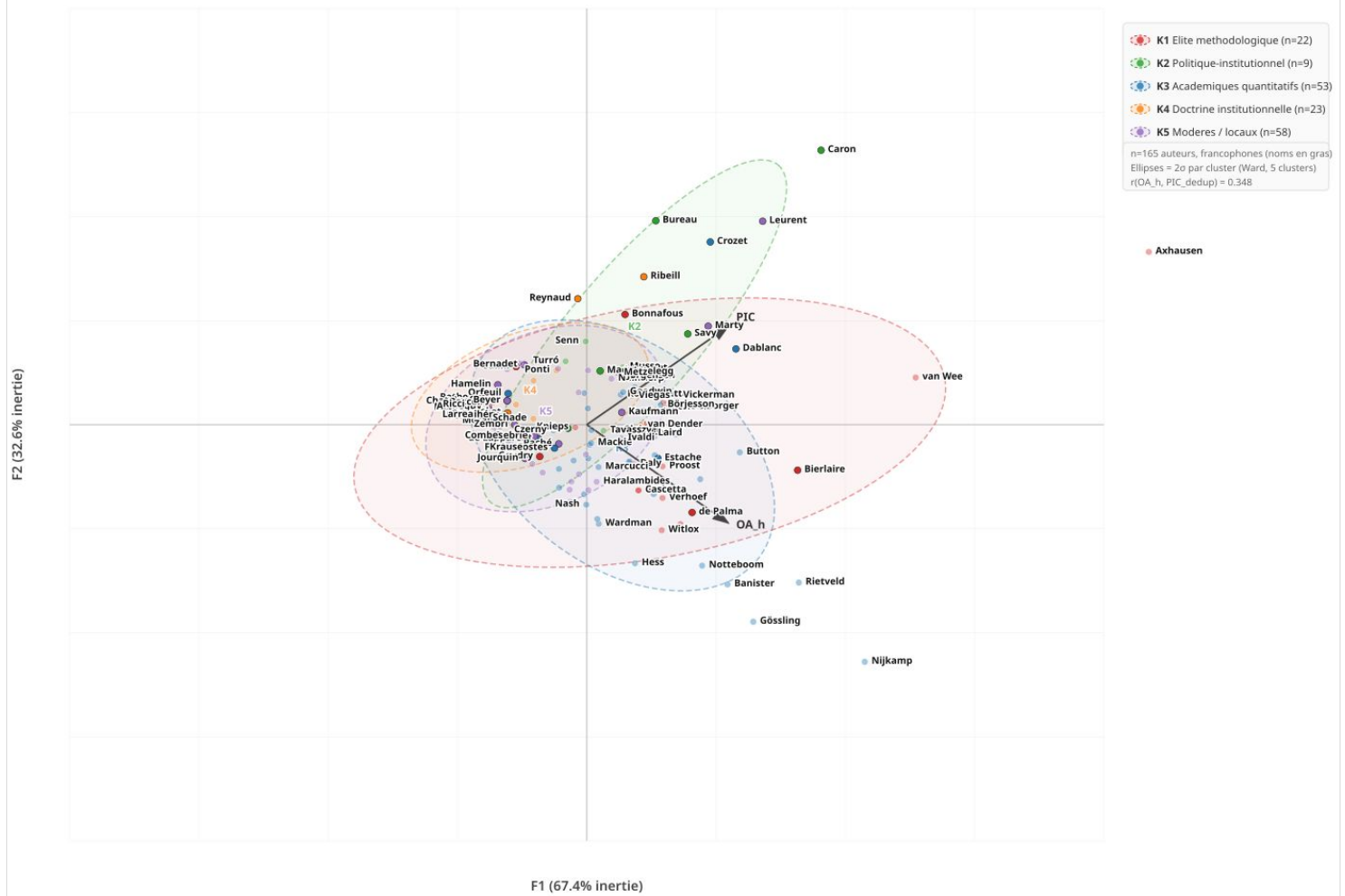
ACP F1 x F2 - PIC_dedup (n=165, Ward K1-K5)
