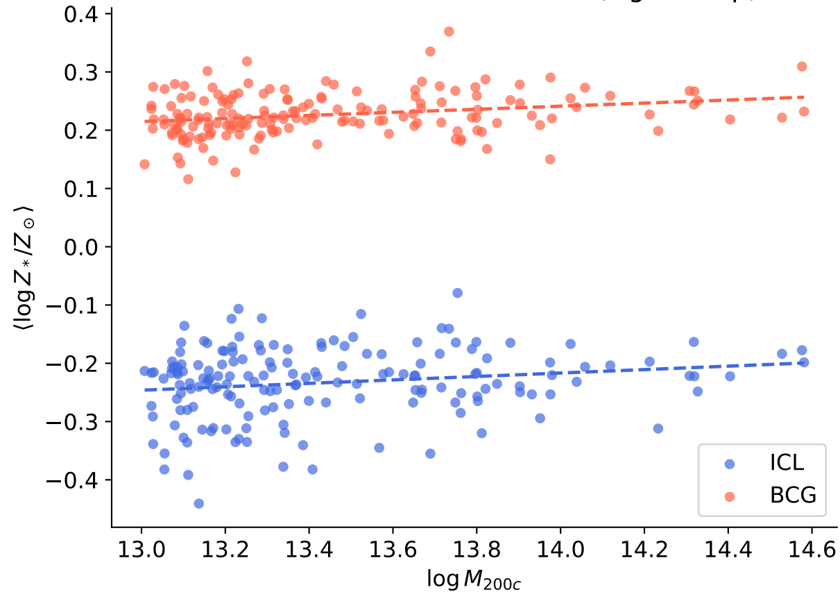
Metallicidad media ICL vs BCG (Fig. 10 top)
