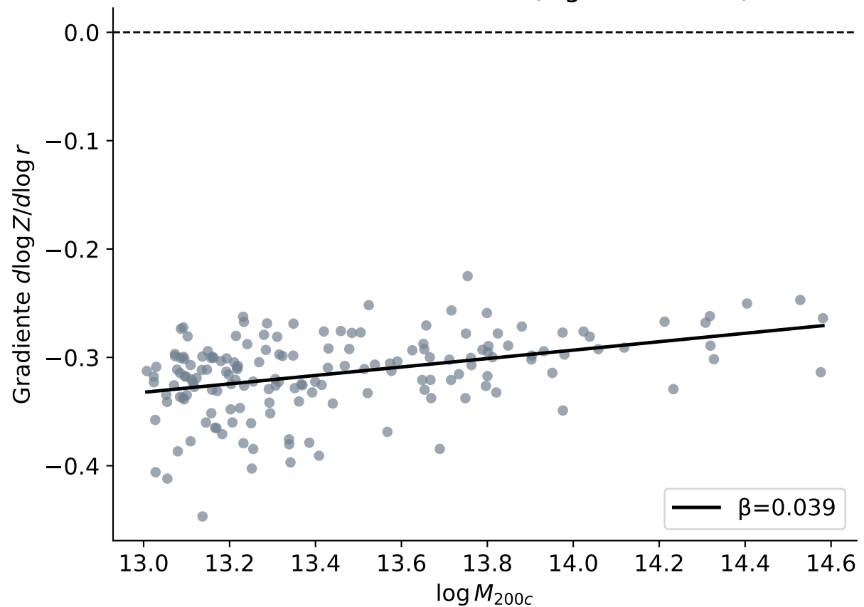
Gradiente metalicidad (Fig. 10 bottom)
