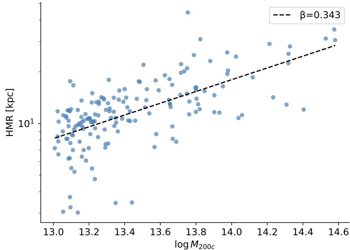
Radio de semi-masa BCG (Fig. 7)
