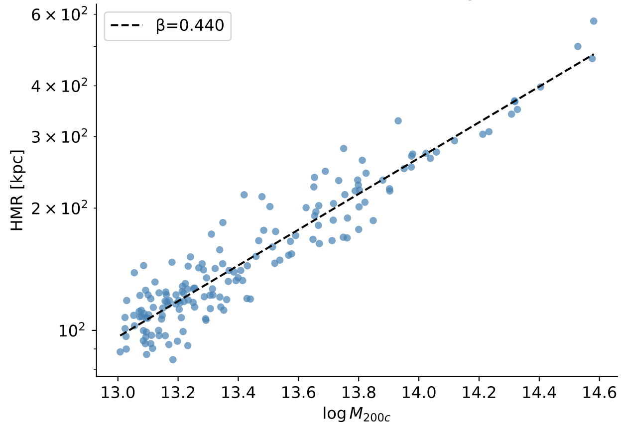
Radio de semi-masa ICL (Fig. 7)
