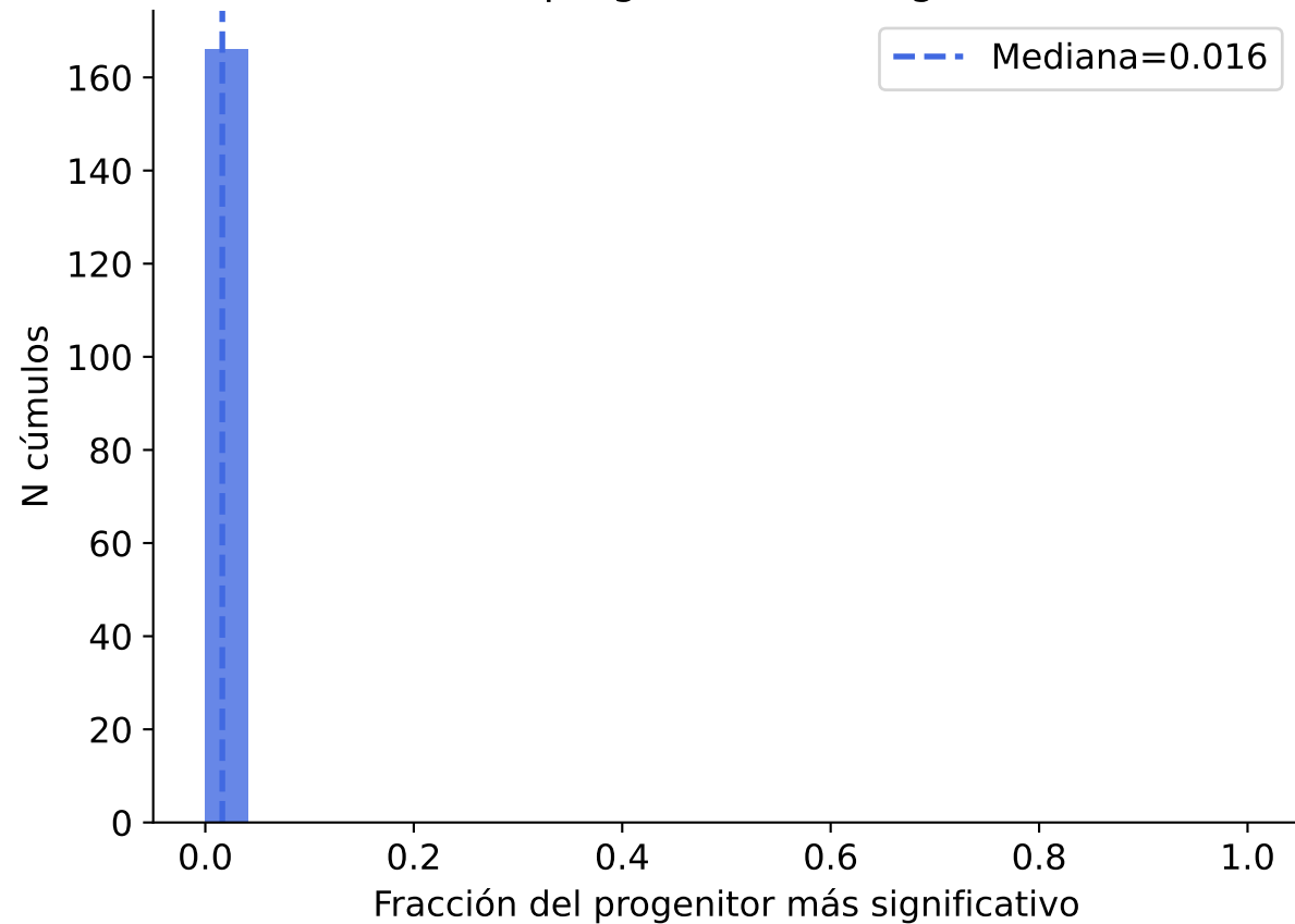
BCG+ICL: progenitor más significativo
