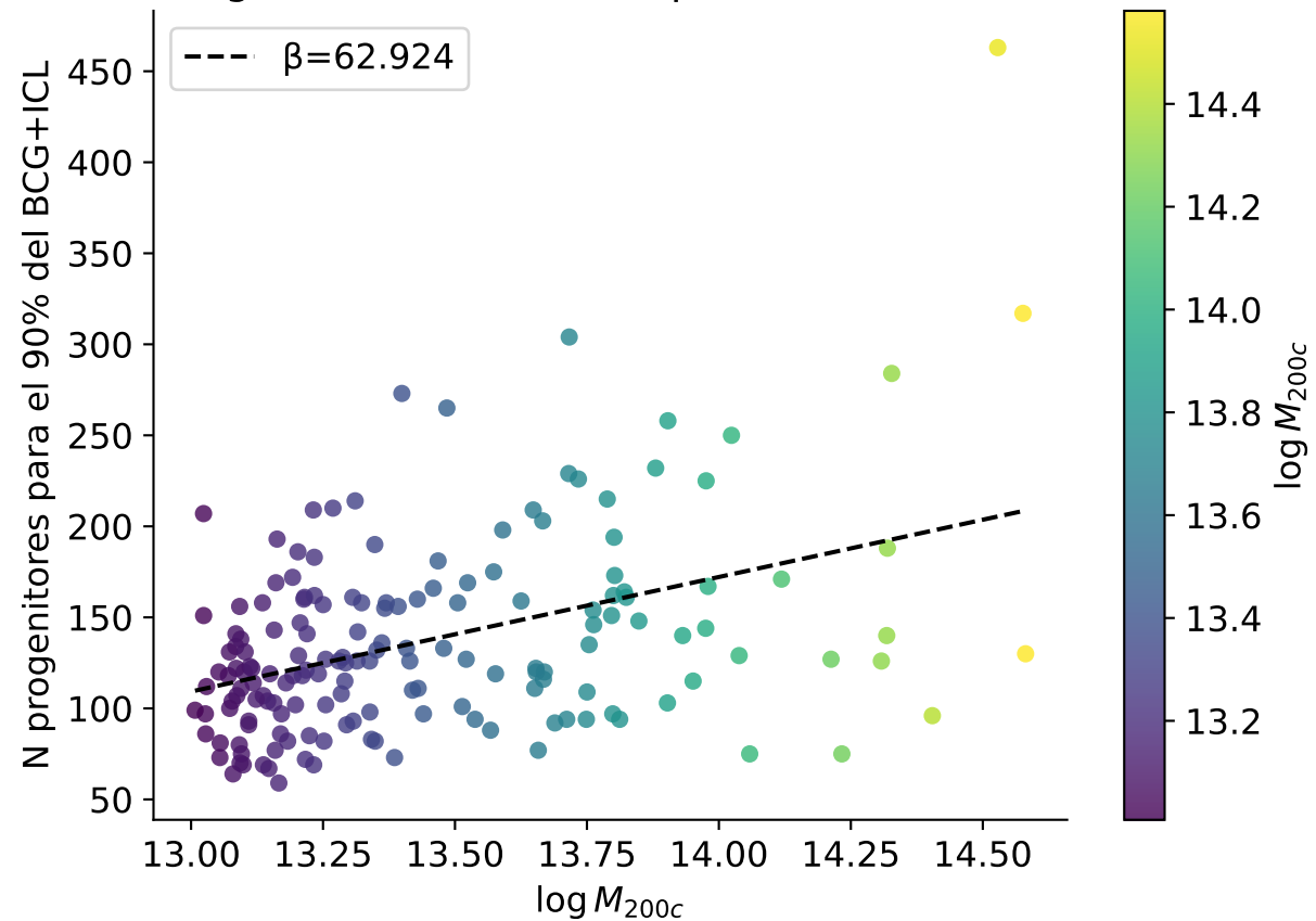
Progenitores necesarios para 90% de masa
