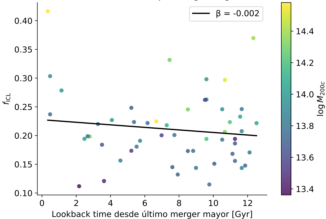
Fracción ICL vs Tiempo merger (Fig. 5)
