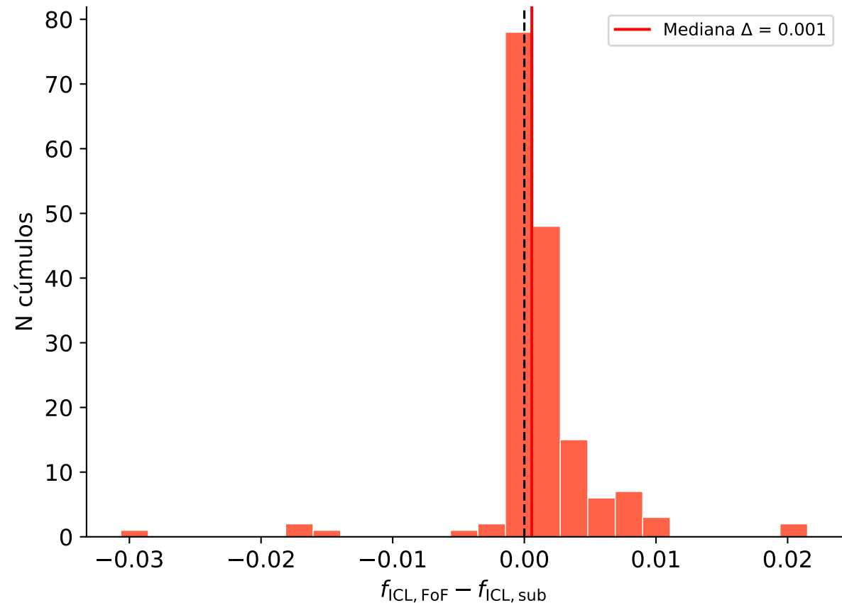
Diferencia FoF – subhalo central
