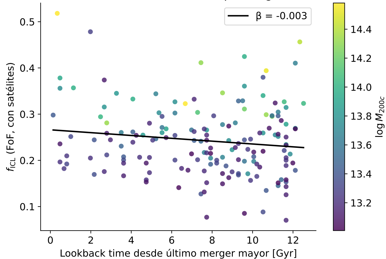
Fracción ICL (FoF) vs Tiempo merger
