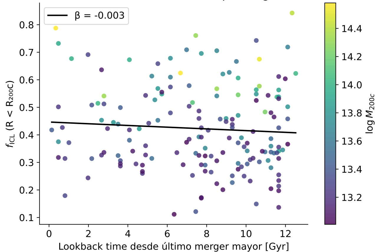
Fracción ICL ( R_{200c} ) vs Tiempo merger
