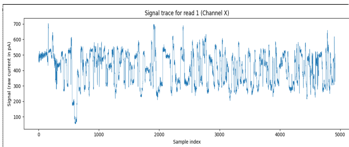
Obr. 1: Príklad surového signálu z nanopore senzoru - signal trace pre jeden kanál. Graf ukazuje elektrický prúd (v pA) meraný v čase počas prechodu DNA molekuly nanopórou.
